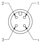
4 PIN M12
