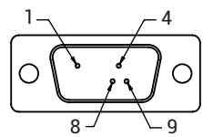
9 PIN DSUB
